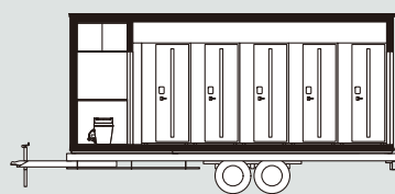
長辺展開図
